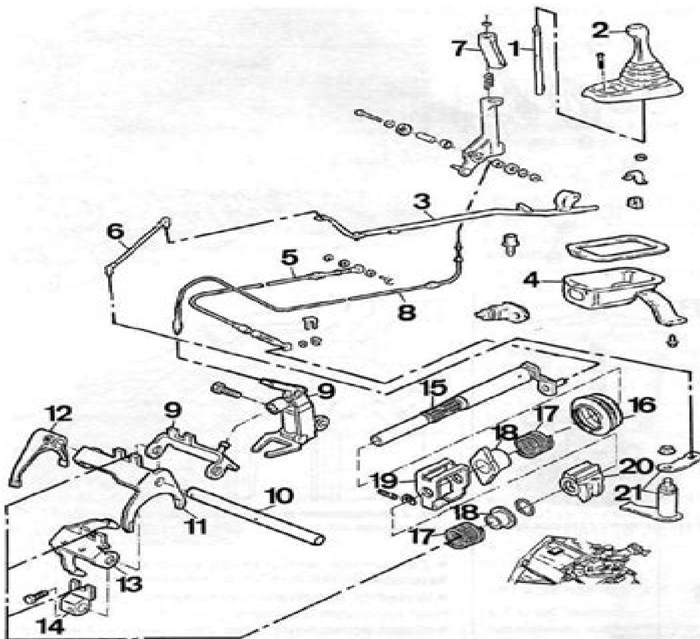
Rys. 4.27. Mechanizm zmiany biegów (skrzynia przekładniowa typu C514) 1 — dźwignia zmiany biegów, 2 — osłona dźwigni zmiany biegów z uchwytem, 3 — drążek podłużny, 4 — obudowa przegubu kulowego dźwigni, 5 — linka sterowania, 6 — łącznik, 7 — dźwignia blokowania biegu wstecznego, 8 — linka wybierania biegu wstecznego, 9 — zespół sterowania z widelkami biegu wstecznego, 10 — osł widełek, 11 — widełki biegów 1—2, 12 — widełki 5. biegu (biegów 5—6 w skrzynce 6-biegowej), 13 — widełki biegów 3—4, 14 — palec sterowania widełek biegów 5—6, 15 — dźwignia sterowania, 16 — osłona, 17 — sprężyny, 18 — tulejki plastikowe, 19 — blokada zabezpieczająca, 20 — palec napędu widełek, 21 — dźwignia wybierania
