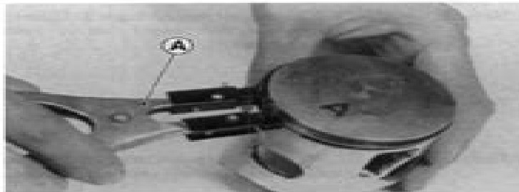
A. Piston Ring Pliers: 57001-115
