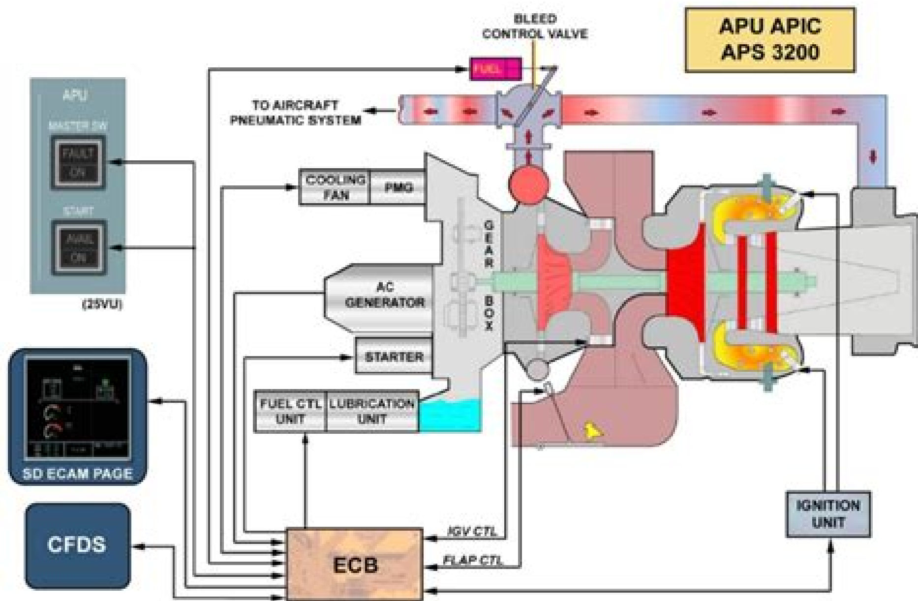
图 1 APS3200 型 APU
