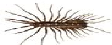
Scutigermorphs
