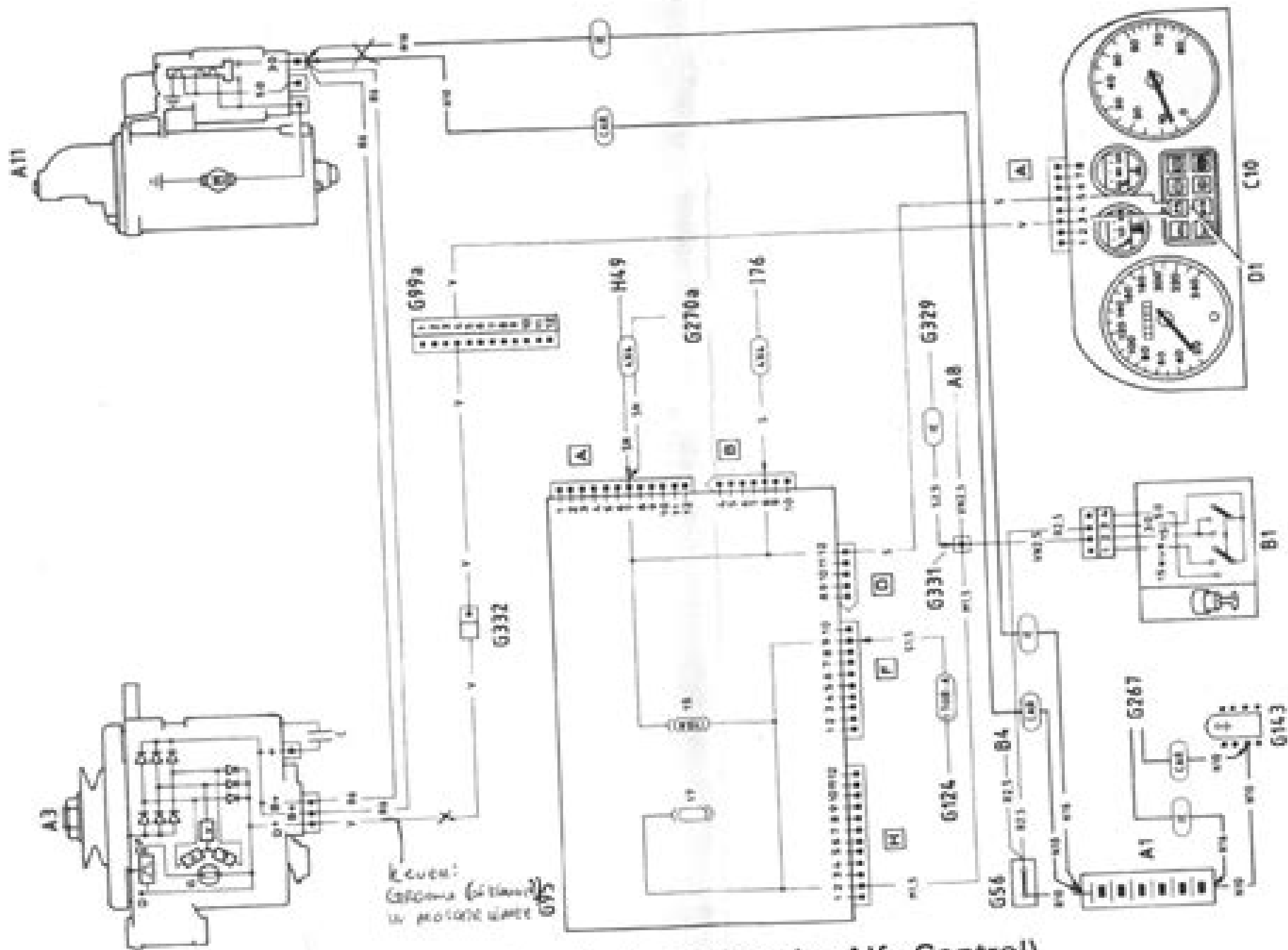
Figuur 12.2: Laadsysteem (zonder Alfa Control)
